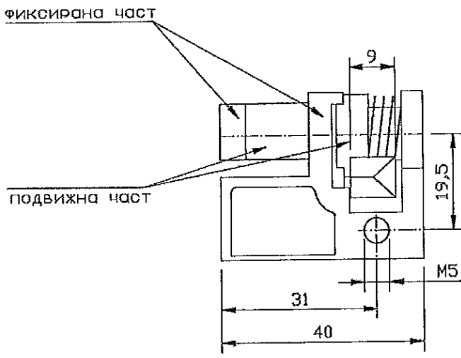
Фигура 1 - Конструкция и размери на галванизирен стоманен ключ и халф цилиндър тип „Полумесец“
